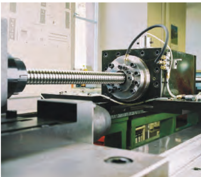
Banco di prova per viti a ricircolazione di sfere
